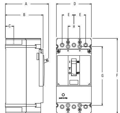
FC 100 Amp Dimensions
