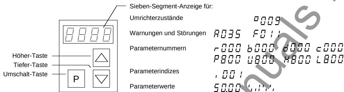
Bild 8-2 Parametriereinheit PMU
