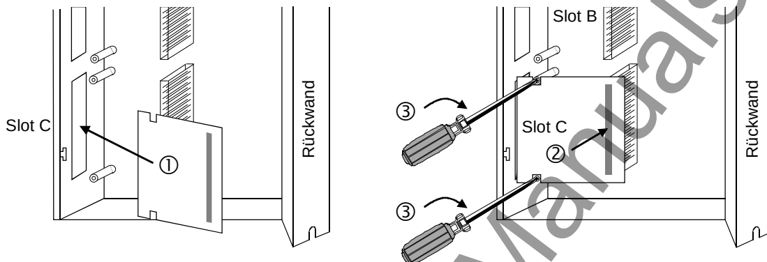
Bild 5-6 Montage der Optionsbaugruppe
