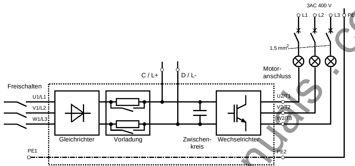
Bild 10-1 Formierschaltung
