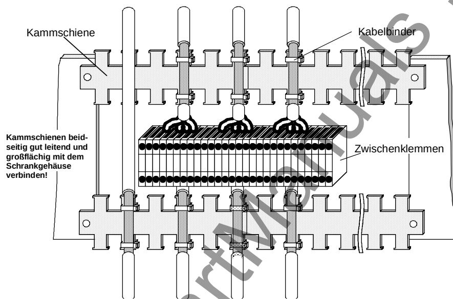
Bild 6-5 Schirmanbindung der Signalleitungen im Schaltschrank
