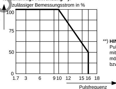
Bild 11-1 Derating-Kurven
