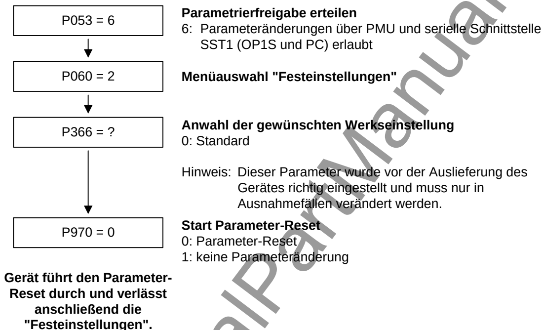
Bild 8-17 Ablauf bei Parameter-Reset auf Werkseinstellung
