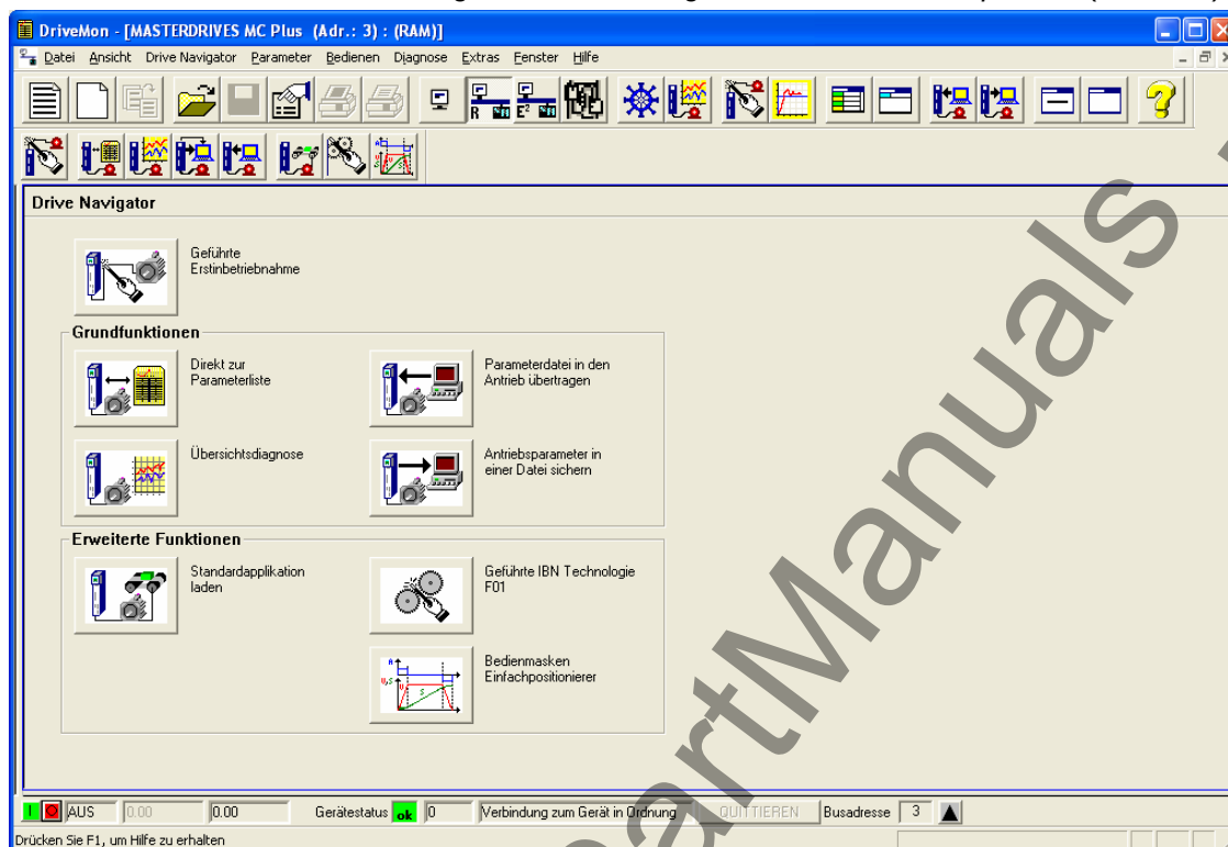
Bild 8-13 Drive Navigator
