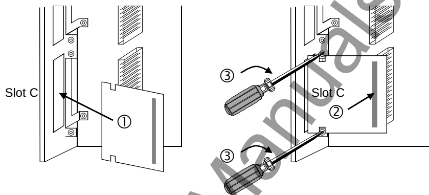
Bild 5-7 Montage der Optionsbaugruppe
