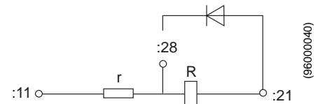
Fig. 2 RXMS 1
