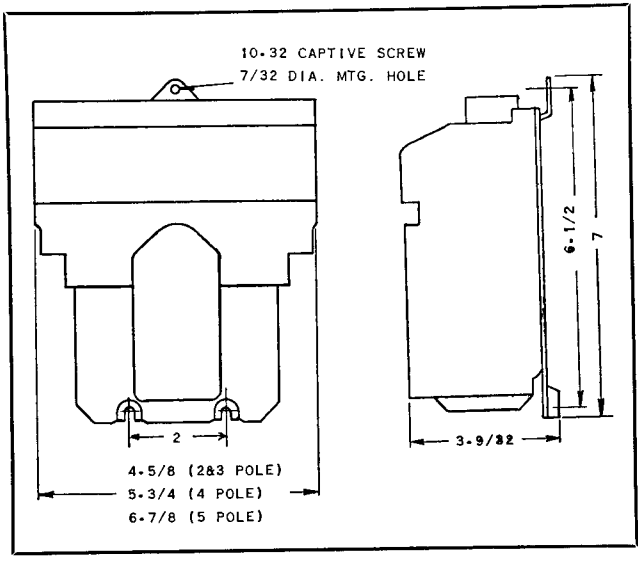
FIG. 3. Size 1—Outline
