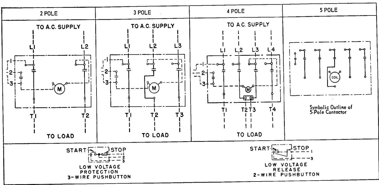
FIG. 2. Wiring Diagram
