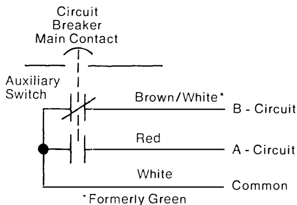
FIG. 38. WIRING DIAGRAM
