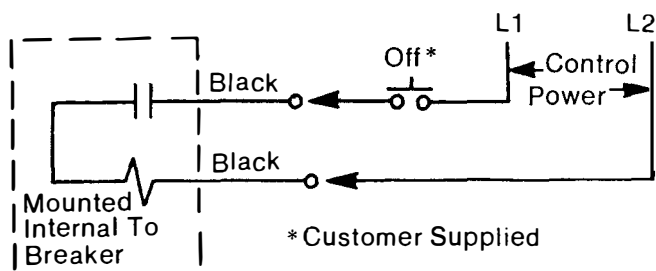
FIG. 22. WIRING DIAGRAM
