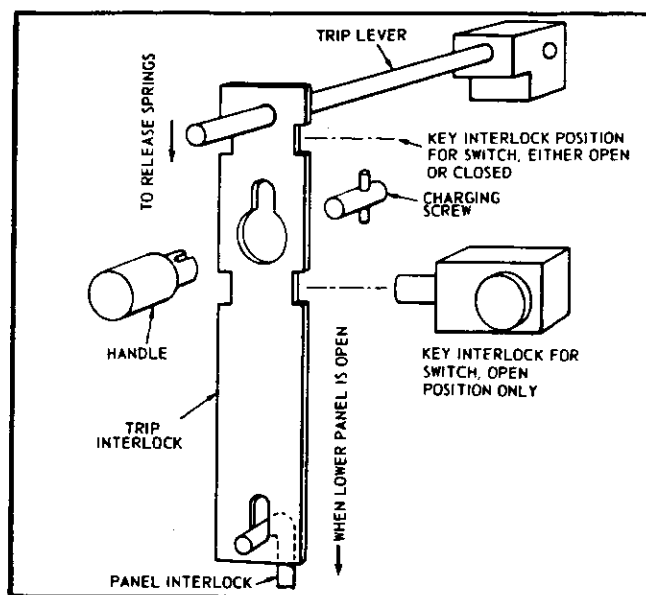
Fig. 26 - Trip interlock.
