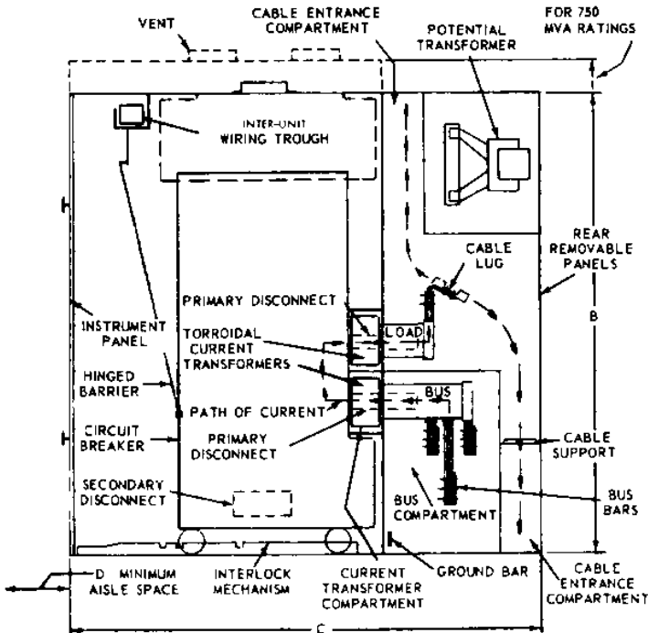
Fig. B — 15-kv Breaker Unit.
