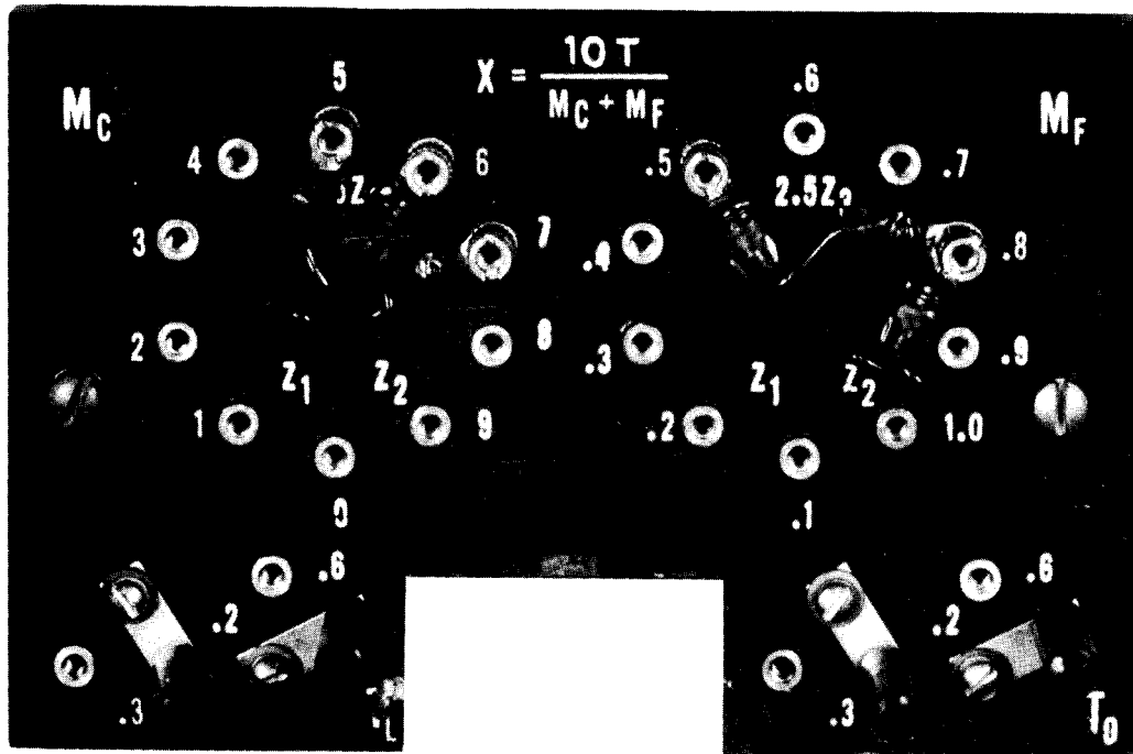
*Fig. 4. Top Plate
