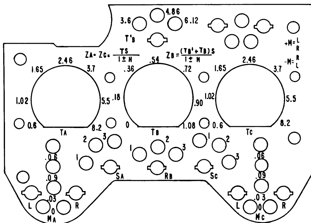
Fig. 6. Tap Plate.
