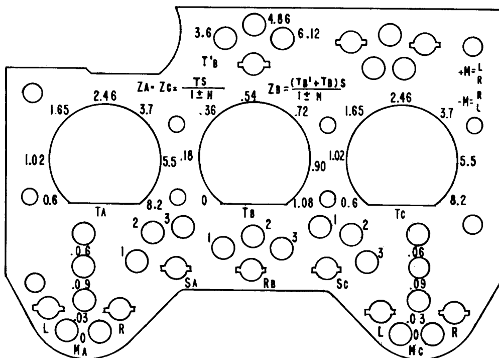
Fig. 6. Tap Plate.
