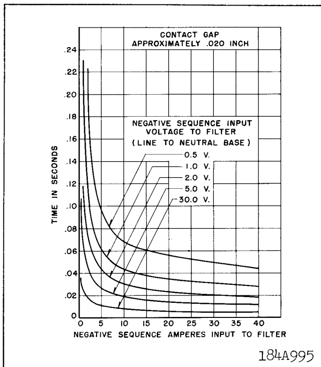
Fig. 6. Time Curve of the Directional Unit (D)
