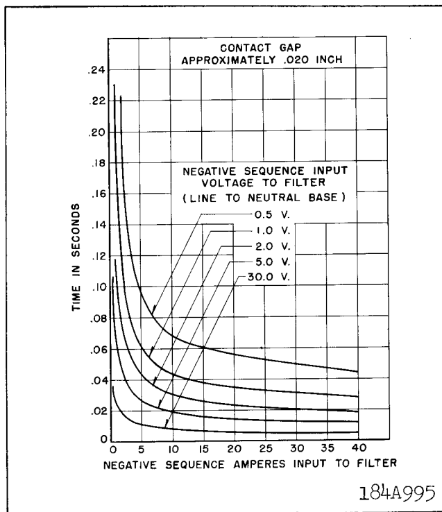
Fig. 6. Time Curve of the Directional Unit (D)
