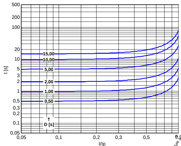
Bild 1-16 Rückfallkennlinie ANSI moderately inverse (M INV)
