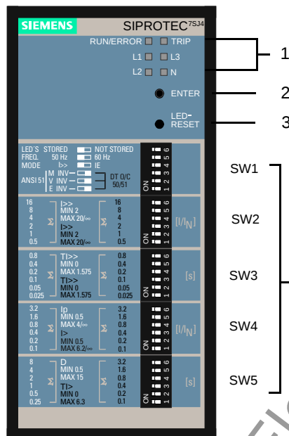
Bild 1-1 Gerätefront Bedien- und Anzeigeelemente des 7SJ46
