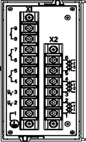
Bild 1-3 Geräterückseite Anschlüsse 7SJ46
