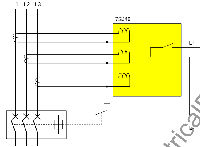
Bild 1-22 Anschluss 7SJ46 bei 3-Wandlerschaltung
