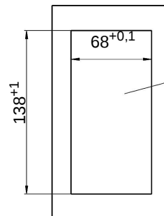
Bild 1-7 Maßzeichnungen
