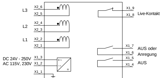
Bild 1-9 Anschlussschaltplan 7SJ46
