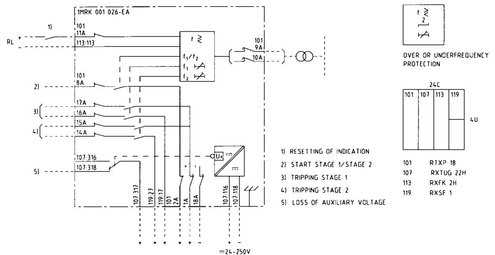
Fig. 2 Terminal diagram 1MRK 001 026-EAA
