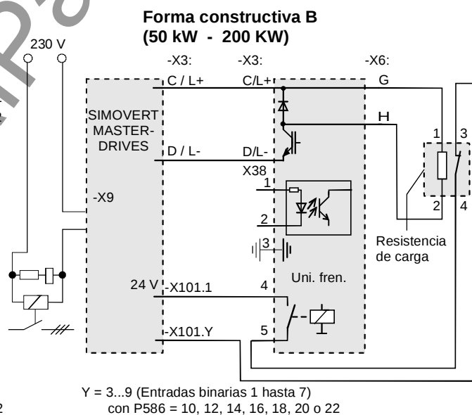
Figura 3-6 Convertidor - Unidad de frenado con resistencia de frenado externa y desconexión por fallo del convertidor
