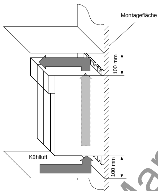
Bild 4-1 Mindestabstände für die Kühlung
