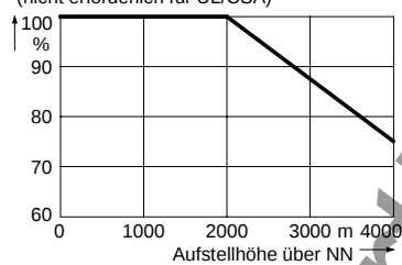
Bild 6-1 Derating
