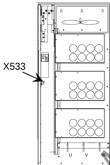
Bild 7-8 Bauformen \geq J
