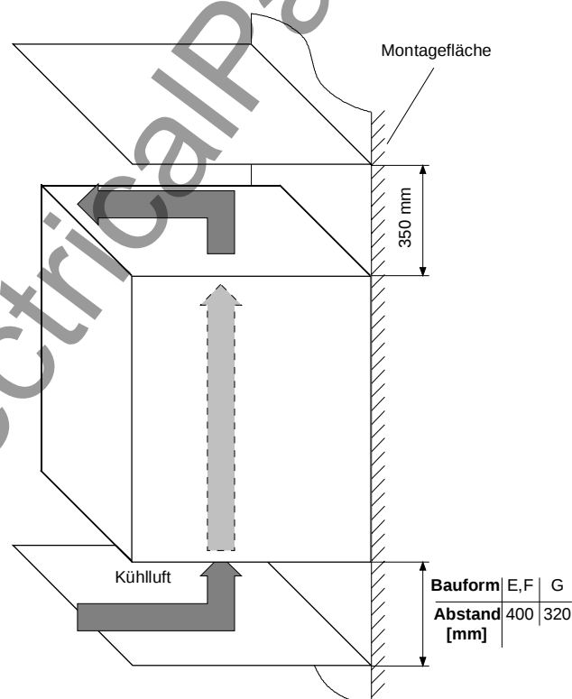
Bild 5-1 Mindestabstände für den Kühlluftbedarf (Bauform E, F, G)
