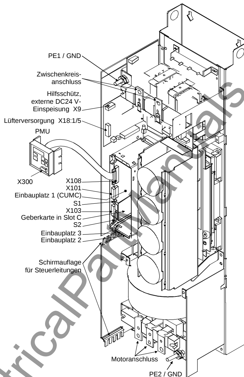
Anschlussübersicht Bauform E und F
