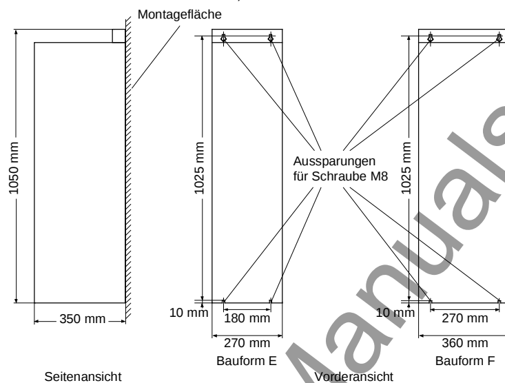
Bild 5-2 Maßbild Bauformen E, F
