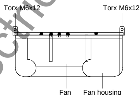
Fig. 9-1 Fan assembly
