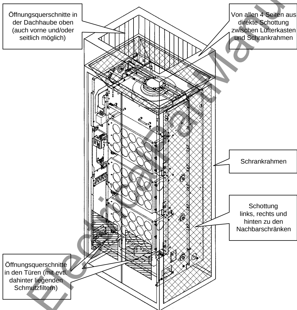
Bild 5-6 Schottungsmaßnahmen
