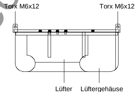
Bild 9-1 Lüfterbaugruppe
