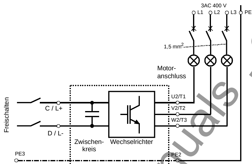
Bild 10-1 Formierschaltung
