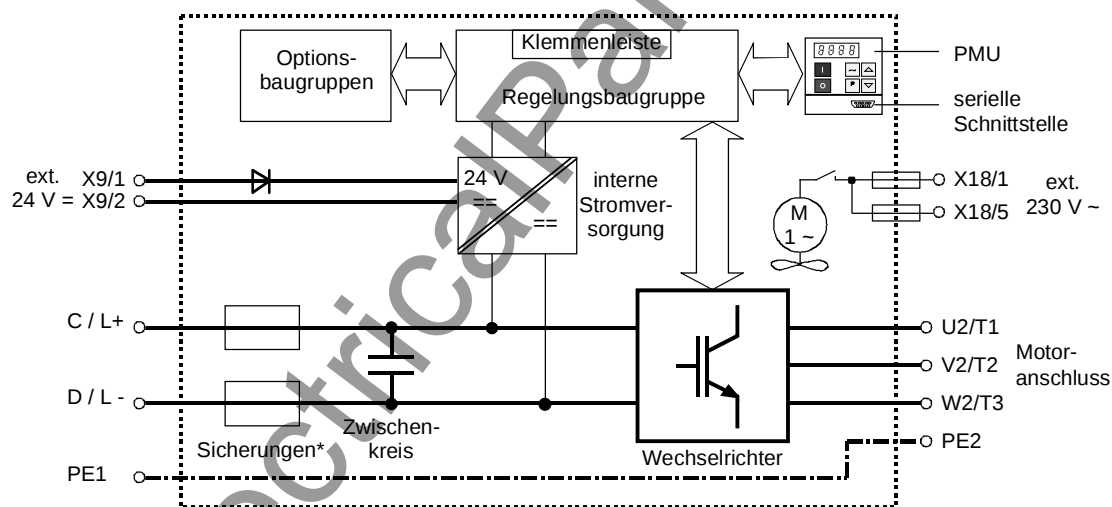
Bild 2-1 Schaltungsprinzip des Wechselrichters
