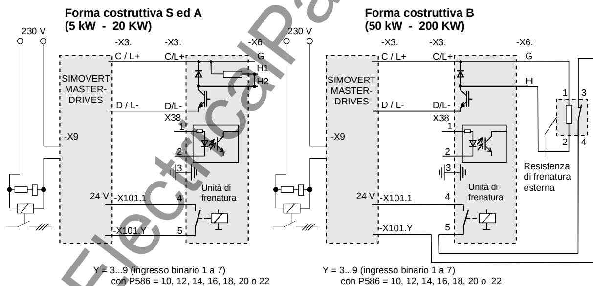
Fig. 3-5 Convertitore - Unità di frenatura con resistenza di frenatura interna e disinserimento per guasto del convertitore
