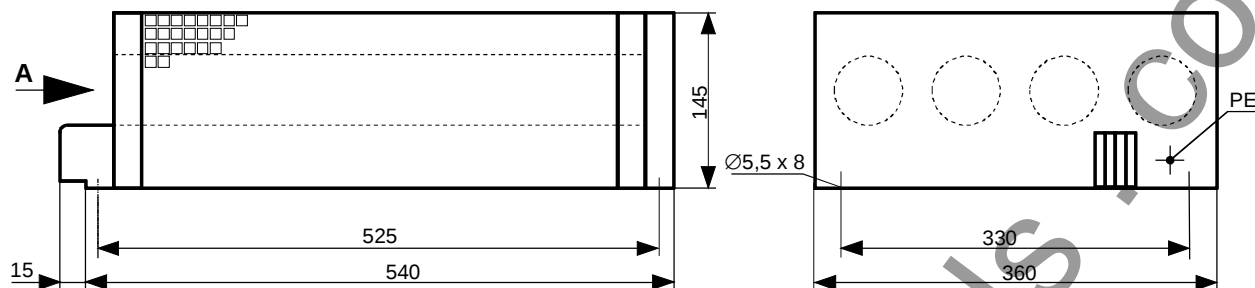
Montaggio tetto armadio
