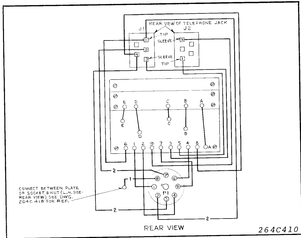
Fig. 8. Wiring Diagram
