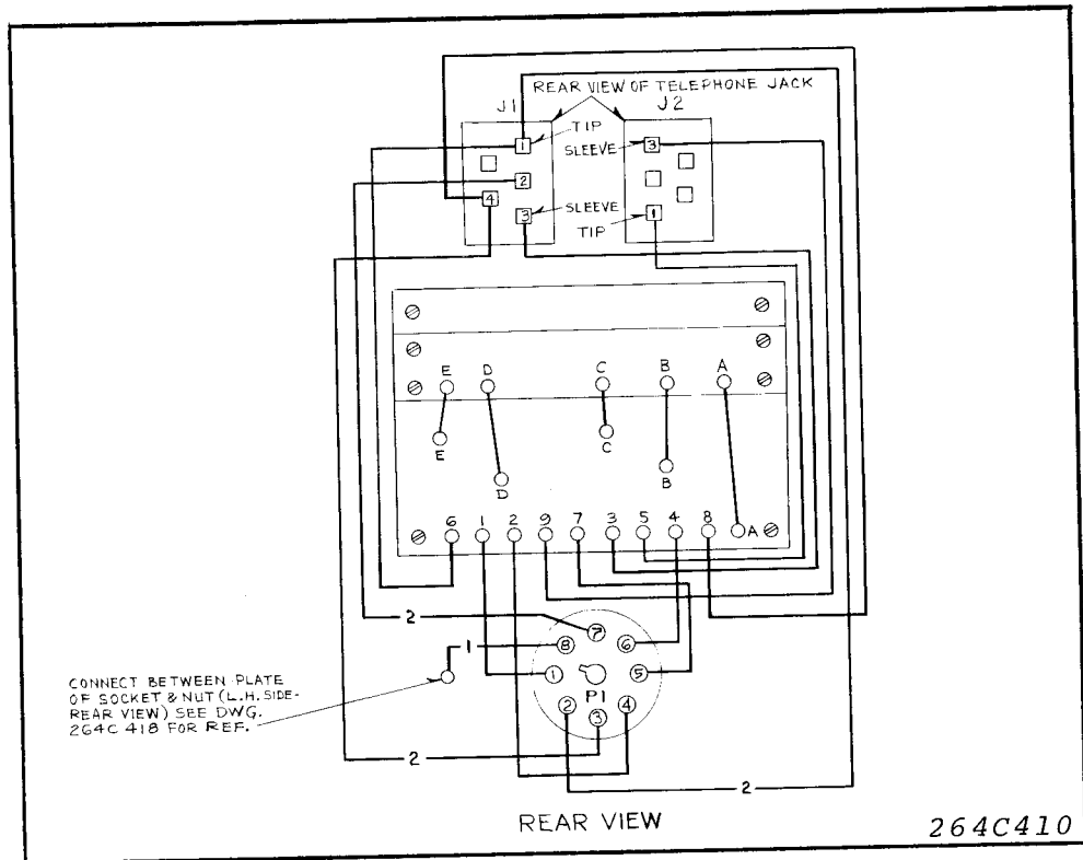
Fig. 8. Wiring Diagram
