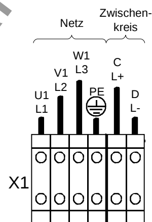
Bild 3.1 Netzanschluß
