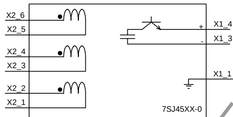
Bild 1-9 Anschlussschaltplan 7SJ45 mit Impulsausgang
