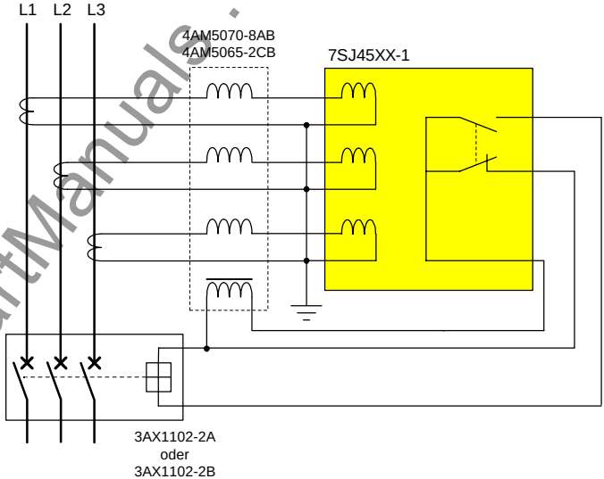
Bild 1-25 3-Wandlerschaltung mit Hilfswandler und Auslöserelais
