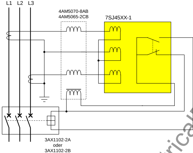
Bild 1-24 2-Wandlerschaltung mit Hilfswandler und Auslöserelais
