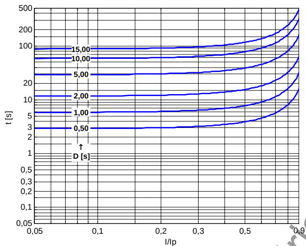
Bild 1-20 Rückfallkennlinie ANSI extremely inverse, (E INV)
