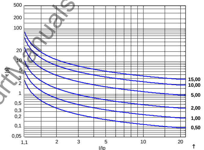
Bild 1-17 Ansprechkenlinie ANSI moderately inverse, (M INV)
