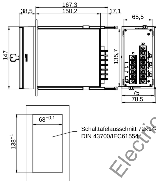
Bild 1-6 Maßzeichnungen
