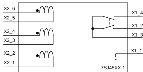
Bild 1-8 Anschlussschaltplan 7SJ45 mit Relaisausgang
