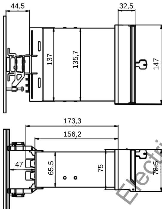
Bild 1-7 Hutschiennenmontage
