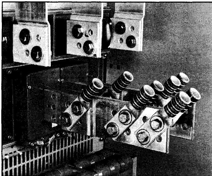
Figure 4-3 Lug Landings
