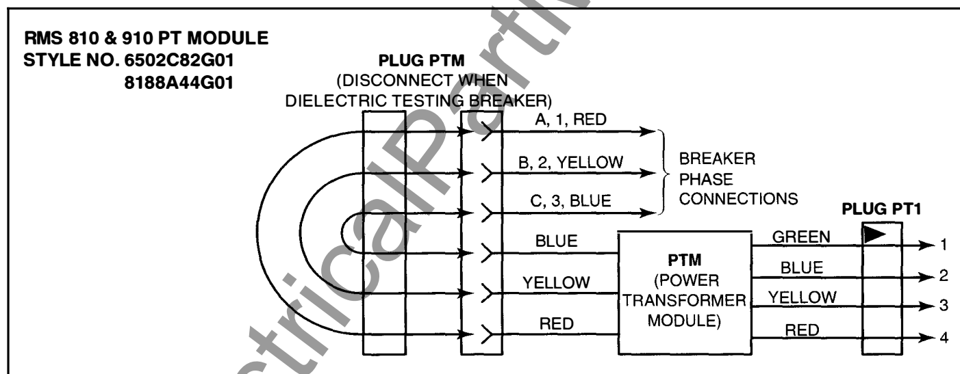
Fig. 12-16 Digitrip RMS 810 &amp; 910 PT Module
